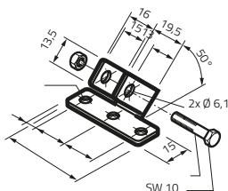
1731901: Raamstoel
