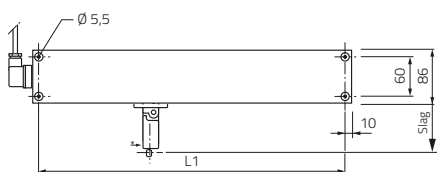
Bovenaanzicht
