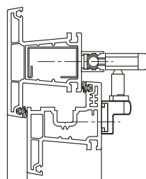
Kunststof kozijn met hoge raamstoel
