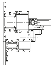
Aluminium kozijn
