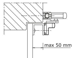
Houten kozijn met verdieptliggende klep
