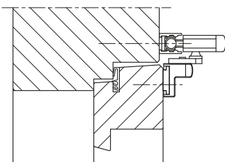
Houten kozijn
